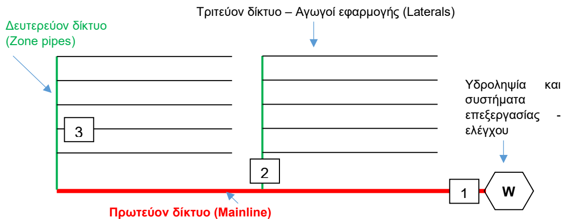
Εικόνα 51 Υδρόμετρο τοποθετημένο στη θέση 1, καταγράφει το 100% της παροχής του συστήματος, τοποθετημένο στη θέση 2 καταγράφει το 50% της παροχής του συστήματος, στη θέση 3 καταγράφει το 10% της παροχής του συστήματος
